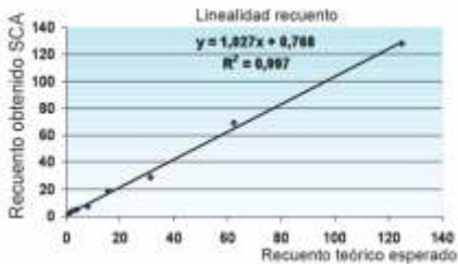
Recuento espermático con SCA, empleando cámara Leja 10, en rango de concentración teórico entre 120 a 0,98 millones/mL. Fig. 3. Intervalo de medición.
